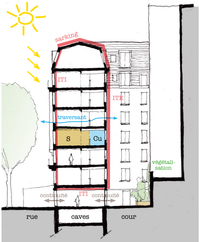
Coupe transversale
