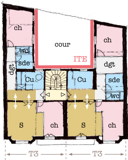
Étage courant
