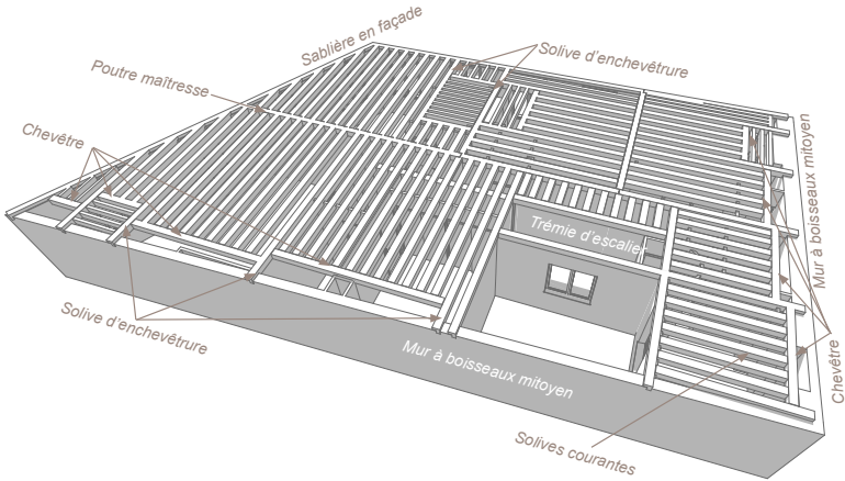
Modélisation structurelle d'un plancher
