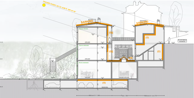
Coupe transversale sur les Ateliers d'artistes
