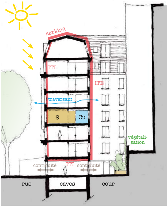
Coupe transversale
